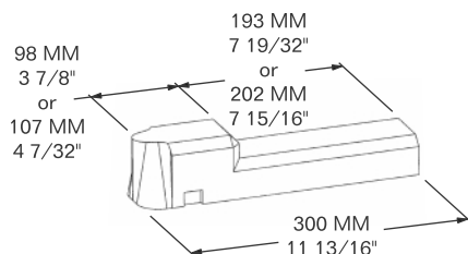
5203-10.71 x 40 - 98 5203-10.71 x 32 - 107 5203-10.71 x 40 - 107 5203-10.94 x 50 - 107 END PIECE
