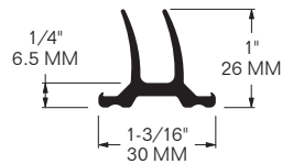
MODEL 1404-6247-A
