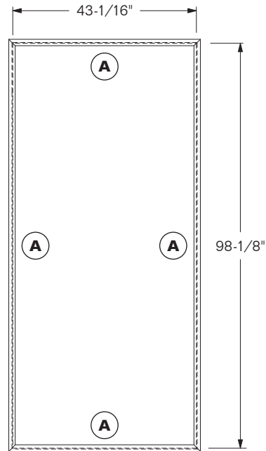
MODEL 1404-6248 THERMAL DOOR GASKET INNER, RIGHT
